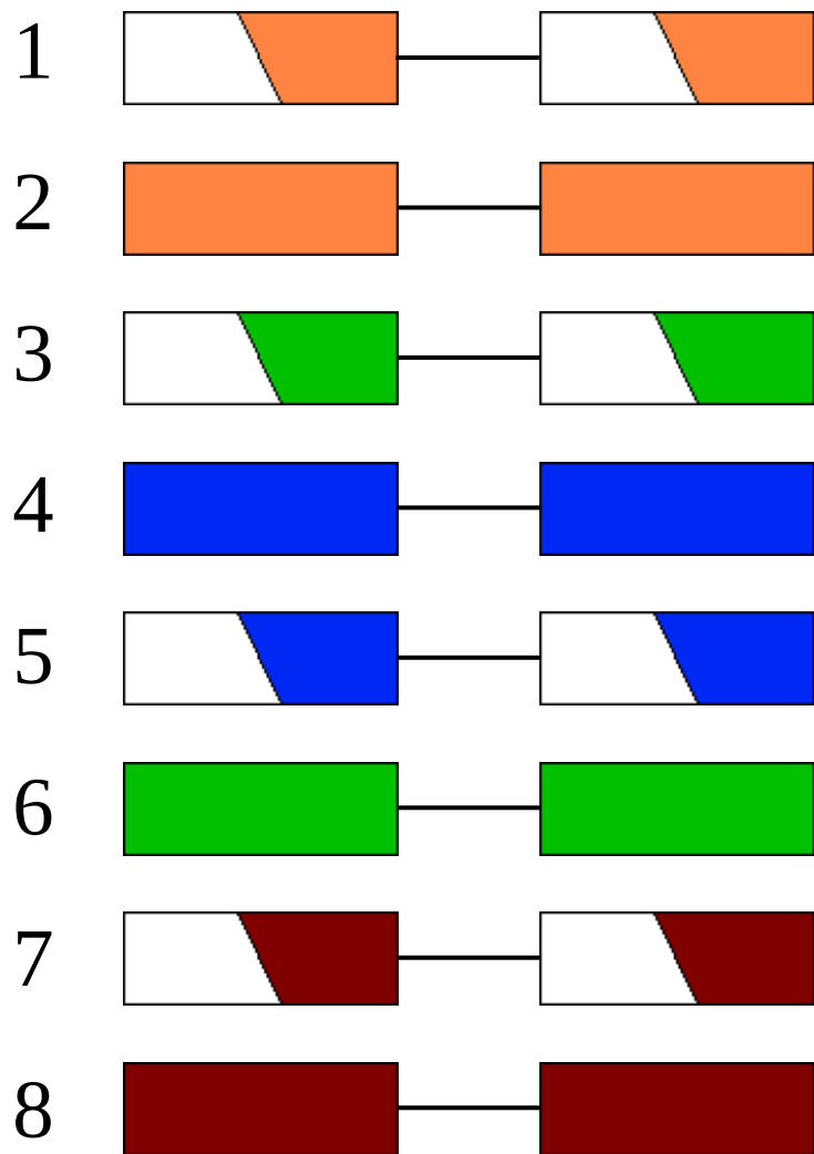
ストレートケーブル
