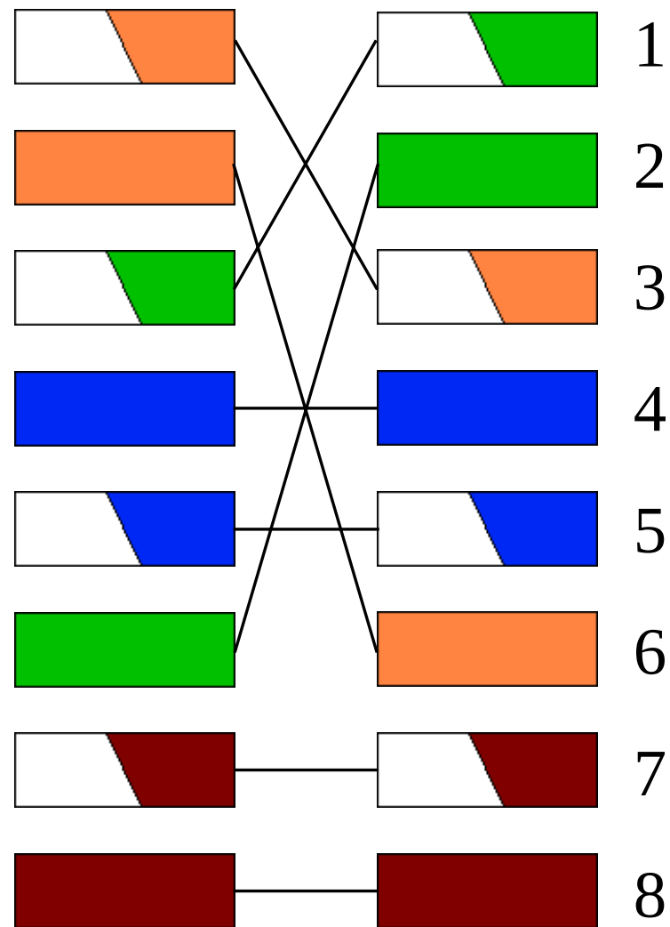
クロスケーブル
